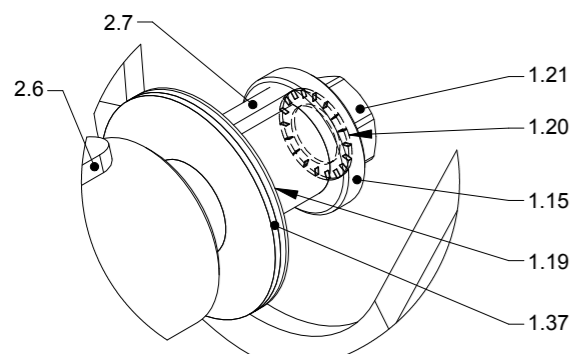
DETAIL B (1 : 2)
