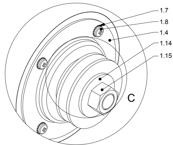
DETAIL B (1 : 2)
